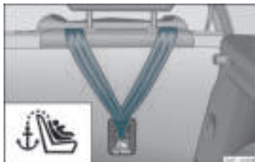
Rys. 27 Oparcia tylnych siedzeń: uchwyty mocujące Top Tether.
