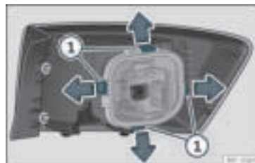
Rys. 48 Zaczepki mocowania na tylnej stronie zespołu światła tylnych.
