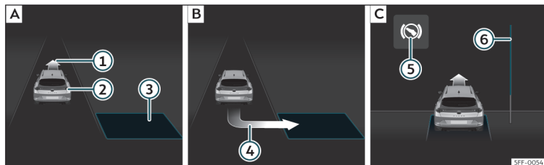
Rys. 173 Na wyświetlaczu tablicy rozdzielczej: parkowanie prostopadłe. [A] Znalazienie miejsca parkingowego. [B] Miejsce do zaparkowania. [C] Manewrowanie.
