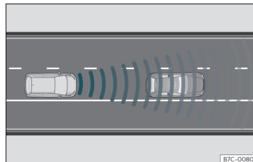
Rys. 141 Obszar wykrywania.
