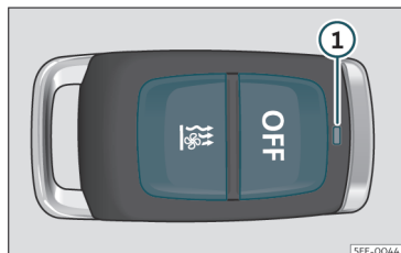
Rys. 125 Ogrzewanie pomocnicze: pilot radiowy zdalnego sterowania.
