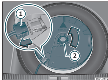
Rys. 198 W bagażniku: wyjąć głośnik niskotonowy. »
