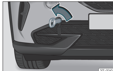
Rys. 44 Prawa strona przedniego zderzaka: pierścień holowniczy na miejscu.
