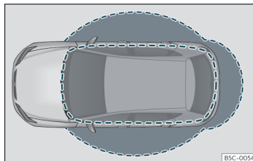
Rys. 72 System Keyless: strefy działania.
