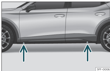
Rys. 38 Punkty unoszenia.
