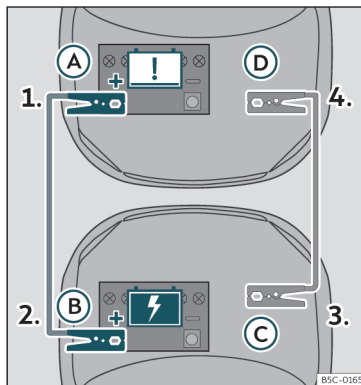
Rys. 42 Schemat połączeń dla pojazdów z systemem Start-Stop.
