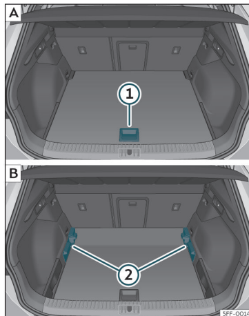
Rys. 109 Regulowana podłoga bagażnika: A pozycja uniesiona; B pozycja obniżona.
