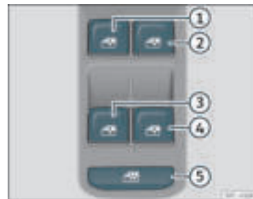
Rys. 91 Szczegółowy widok drzwi kierowcy: przyciski sterowania szybami.
