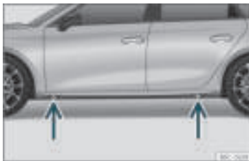
Rys. 42 Punkty unoszenia.
