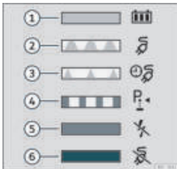
Rys. 204 Po wewnętrznej stronie klapki gniazda ładowania: naklejka z opisem wskaźnika procesu ładowania.
