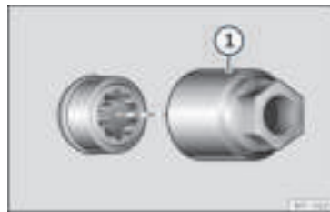
Rys. 40 Śruba przeciwnakradzieżowa do koła z nasadką i adapterem.
