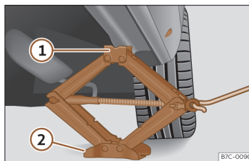
Rys. 236 Belka poprzeczna: ustawianie podnośnika pod pojazdem.
