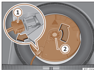
Rys. 231 W bagażniku: wyjmowanie głośnika niskotonowego.
