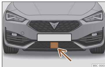
Rys. 121 Na przednim zderzaku: czujnika radarowe.
