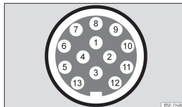
Rys. 194 Schemat: opis styków w gnieździe elektrycznym przyczepy.
